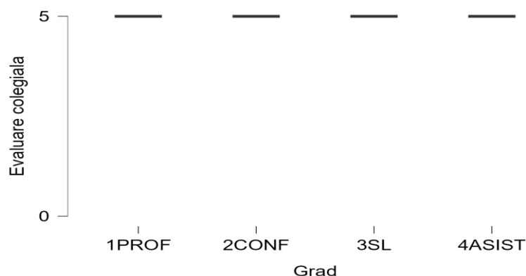
Figura 5. Diagrama boxplot aferentă punctajelor obținute de cadrele didactice la evaluarea colegiala
