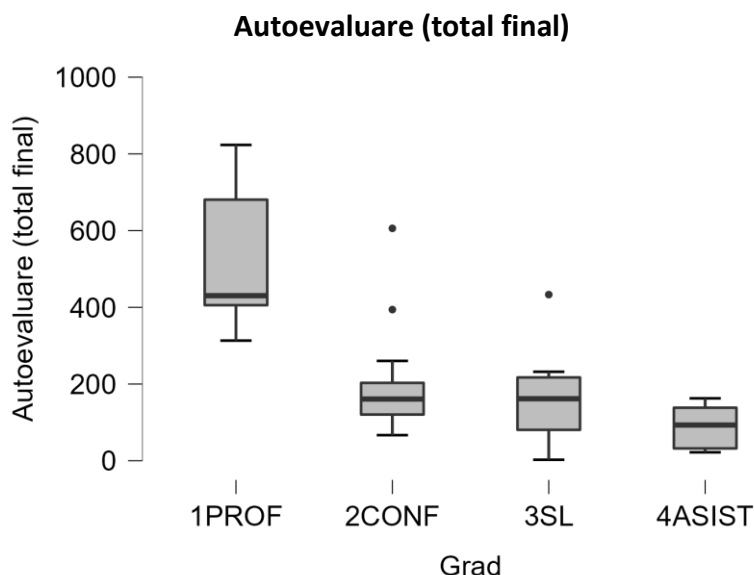
Figura 3. Diagrama boxplot aferentă punctajelor obținute de cadrele didactice la autoevaluare (punctaj total final)
