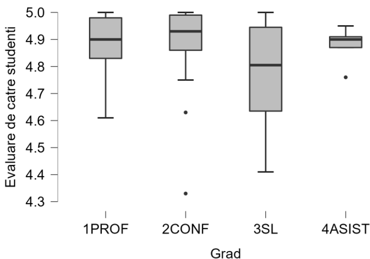
Figura 4. Diagrama boxplot aferentă punctajelor obținute de cadrele didactice la evaluarea de către studenți
